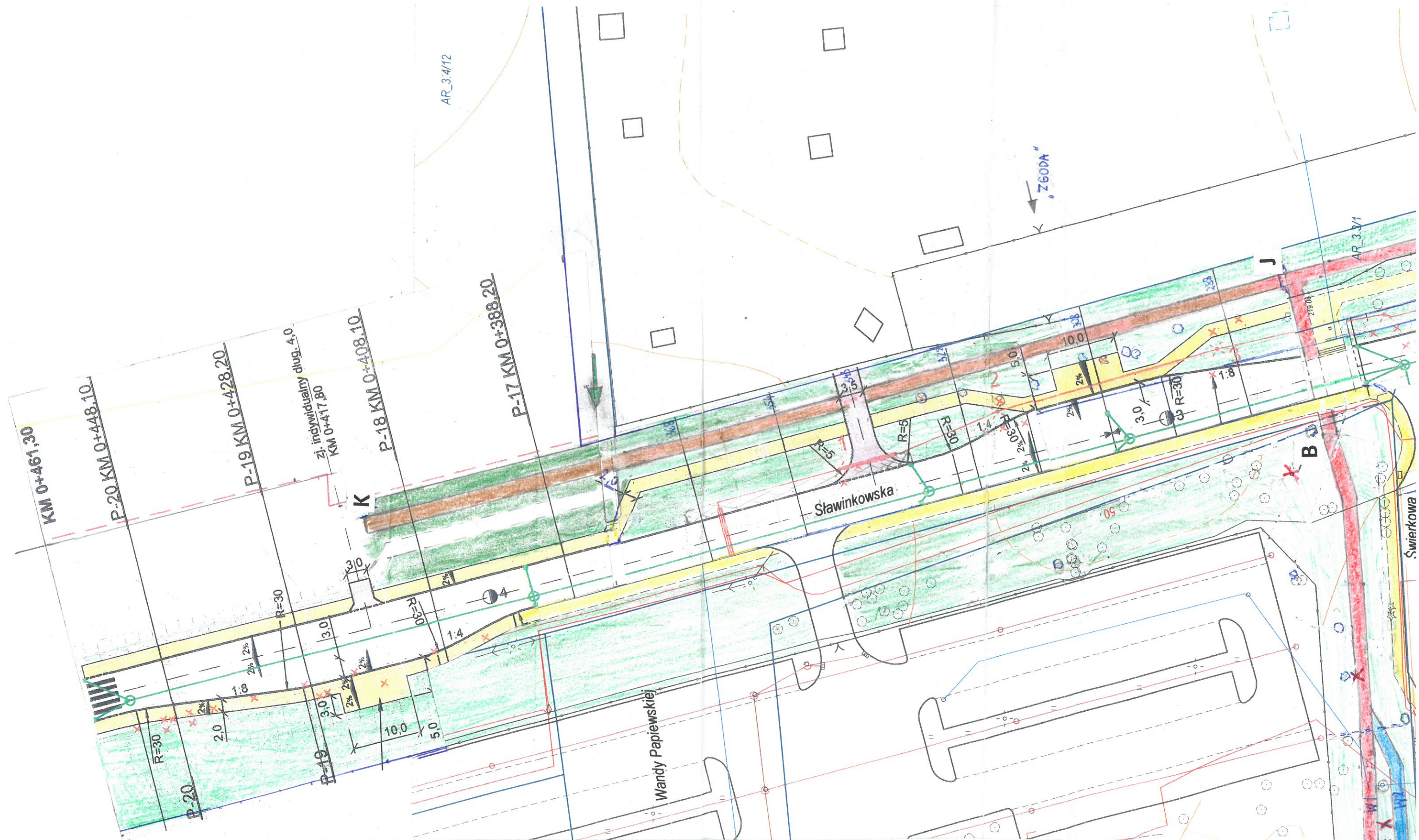
RYS. nr 5 BUDOWA ŚCIEŻKI ROWEROWEJ WZDŁUŻ UL. SŁAWINKOWSKIEJ OD UL. ŚWIERKOWEJ DO PLANOWANEJ DROGI SERWISOWEJ - ODCINEK J-K
