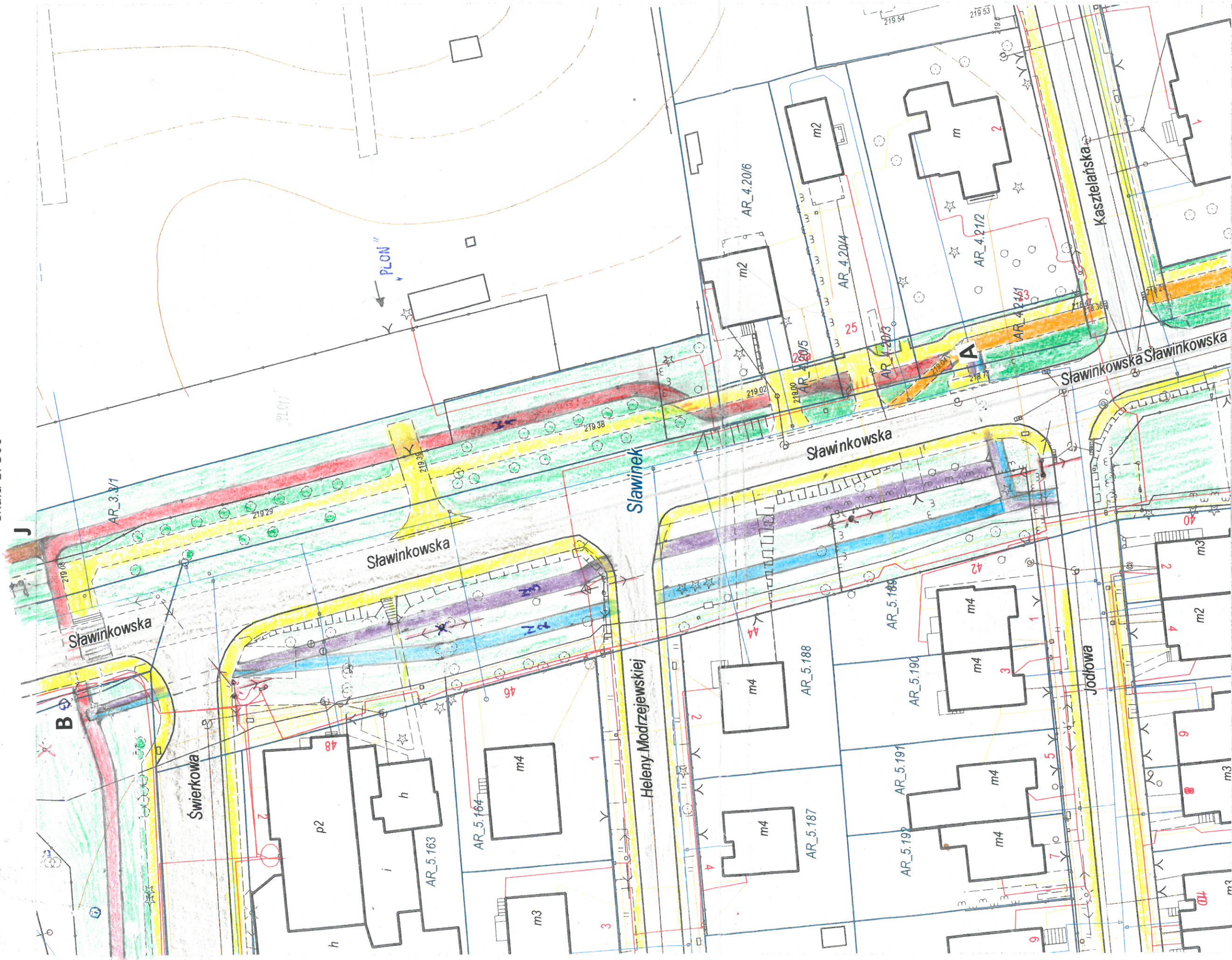
RYS. nr2 KONTYNUACJA BUDOWY ŚCIEŻKI ROWEROWEJ WZDŁUŻ UL. SŁAWINKOWSKIEJ ODCINEK OD UL. JODŁOWEJ DO UL ŚWIERKOWEJ - ODCINEK A-B.
